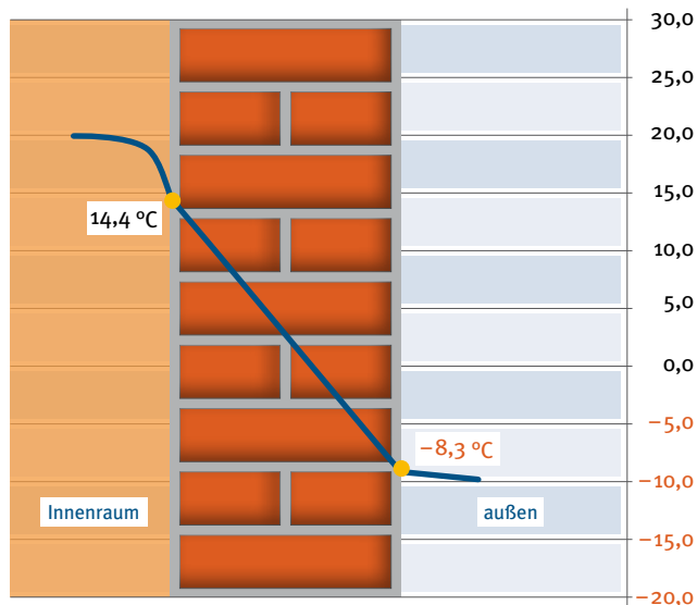
TEMPERATURVERLAUF IN DER AUSSENWAND [°C]
